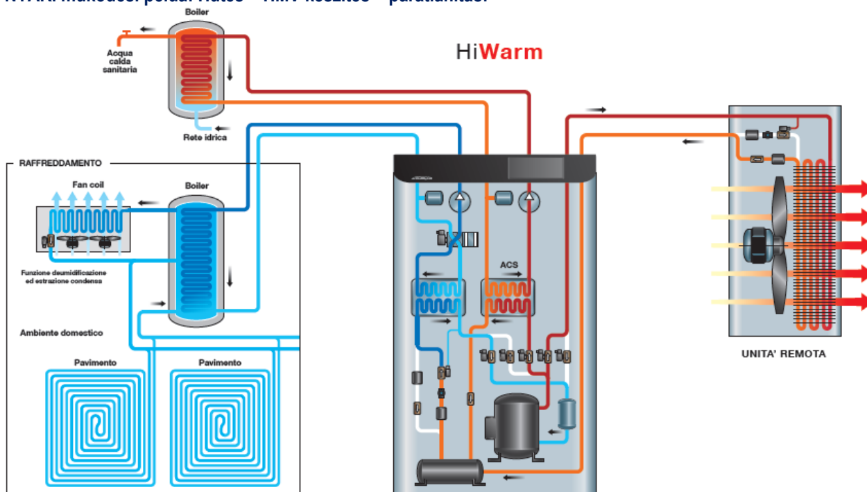
kapcsolási példa Galletti HIWARM teljes hővisszanyeréses berendezésre
