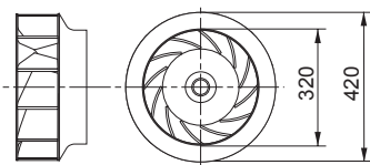
Old fan (13 blades)
