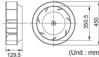
New fan (7 blades)
