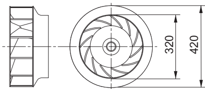
(Unit : mm)
